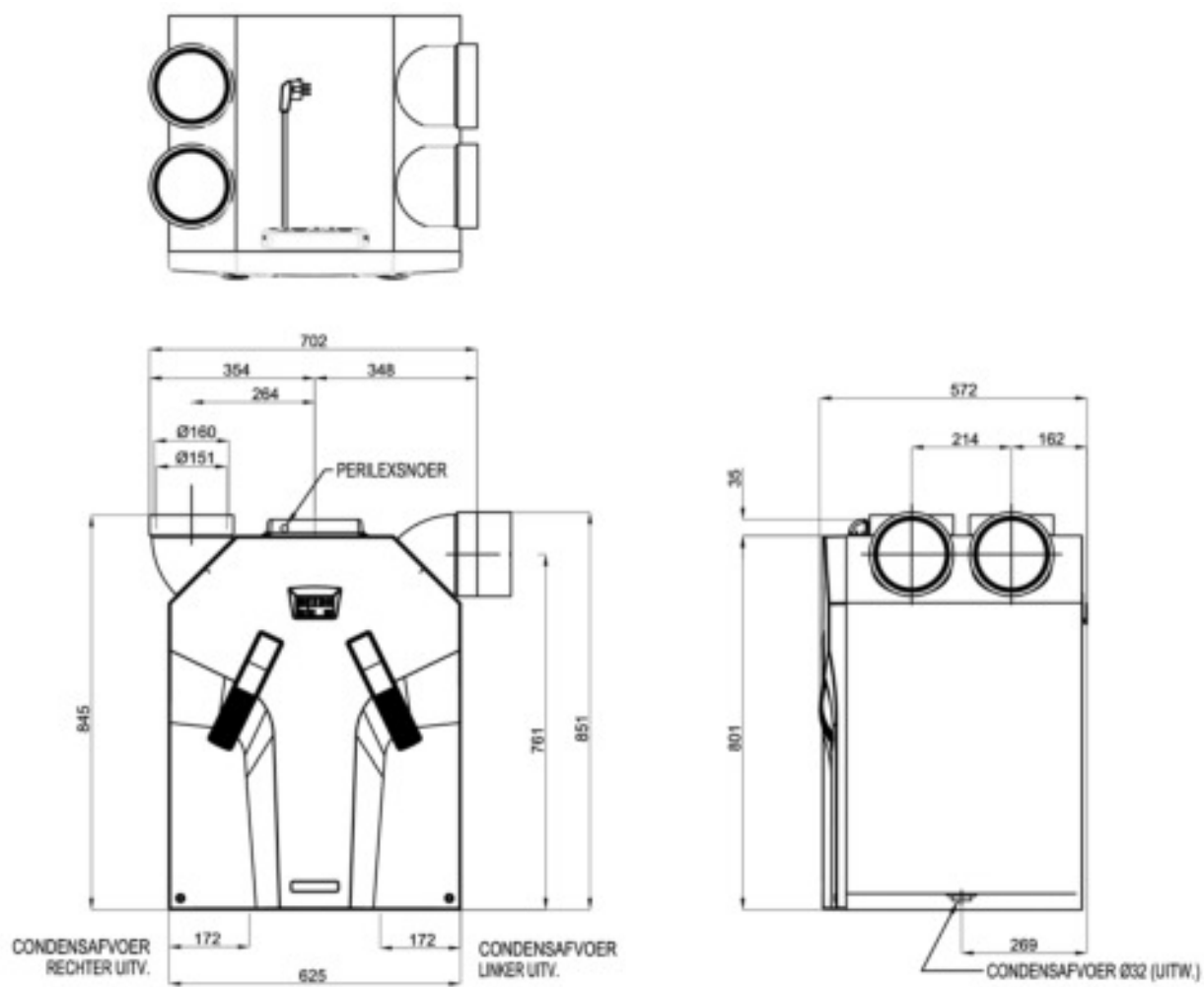
Afbeelding 6.0: Maatschets WHR 930
