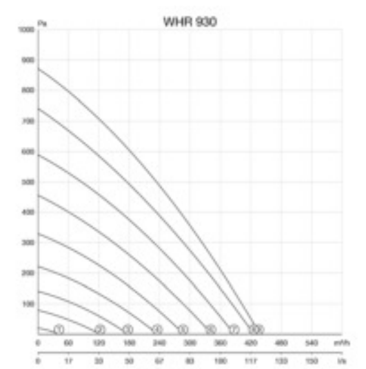
Afbeelding 7.0: Luchtgrafiek WHR 930
